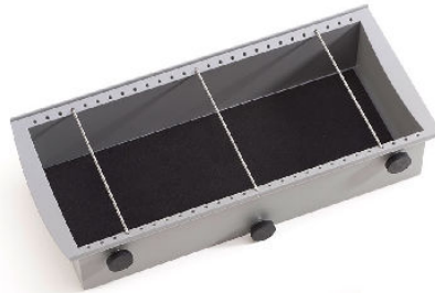
BOITE MAGNETIQUE avec 3 aimants caoutchouc avec caoutchouc antidérapant 345(l)x160(p)x70(h)mm 240.99-21151
