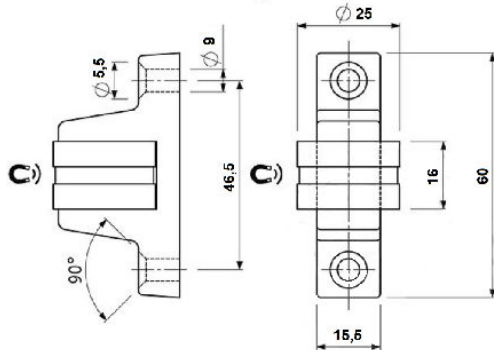
240.99-B60 150N - 60°C - 71g
