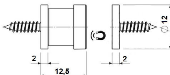
240.99-B12 6N - 60°C - 12,5g
