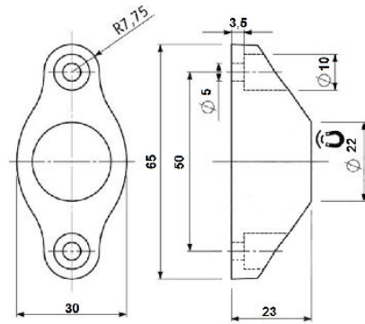
240.99-B65 60N - 60°C - 22g
