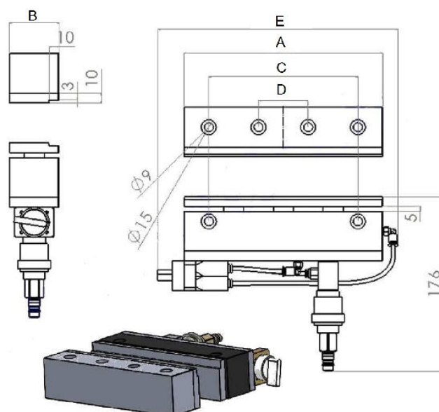
Mors étages lisses 233.99PNPS-150/200-ML épaisseur: 10 mm
